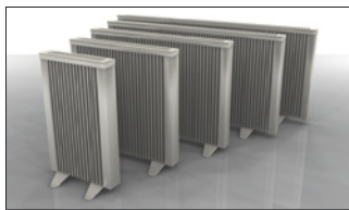
S-Serie: Lässt sich wegen ihrer geringen Tiefe und standardisierten Höhe bequem unterhalb der Fensterbank montieren. Bauhöhe: 63 cm/Tiefe: 8 cm/Leistung: 0,5-3 KW
