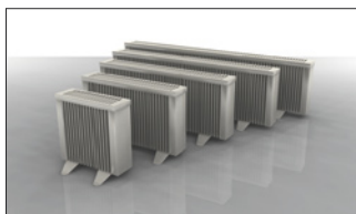
ND-Serie: Perfekt für Räume mit tiefen Dachschrägen oder geringer Brüstungshöhe. Bauhöhe: 38 cm/Tiefe: 13 cm/Leistung: 0,5-2,5 KW
