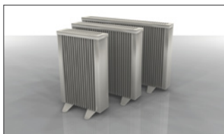
D-Serie: Durch die doppelte Schamotteschicht bringen die Geräte große Leistung und das auf kleinstem Raum. Bauhöhe: 63 cm/Tiefe: 13 cm/Leistung: 1-3 KW
