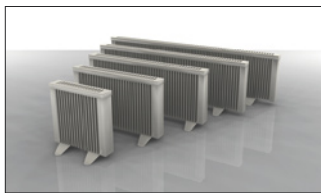
N-Serie: Für Montagen unterhalb von Dachschrägen oder in Räumen mit geringer Brüstungshöhe. Bauhöhe: 38 cm/Tiefe: 8 cm/Leistung: 0,5-2,5 KW
